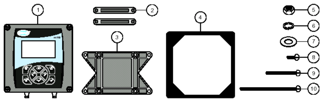
图 2 控制器安装部件
